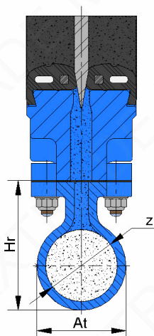
SECCIÓN B-B
