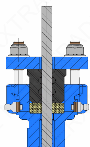
SECCIÓN F-F
